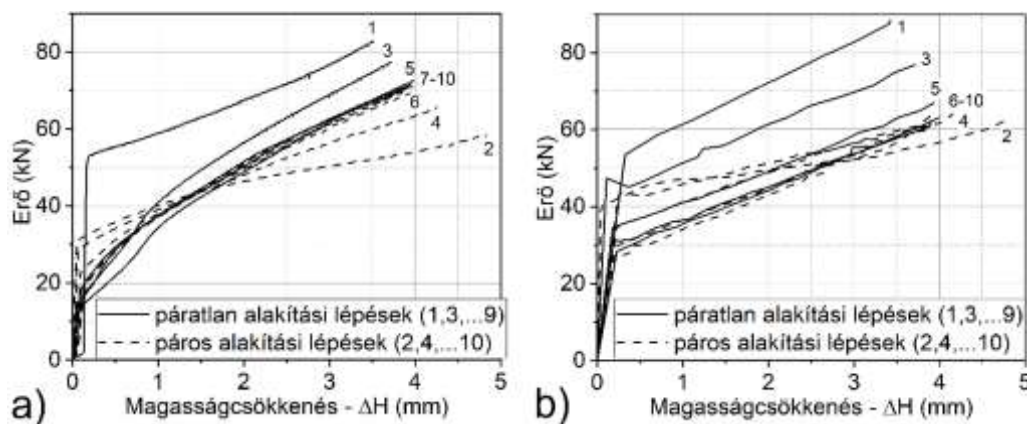
2. ábra. Az erőlefutás a munkadarab magasságcsökkenésének függvényében a fizikai (a) és a végeleemes (b) szimulációban.
