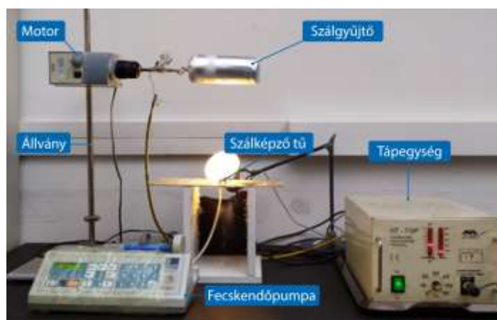
1. ábra. Az alkalmazott elektro-szálképző berendezés
