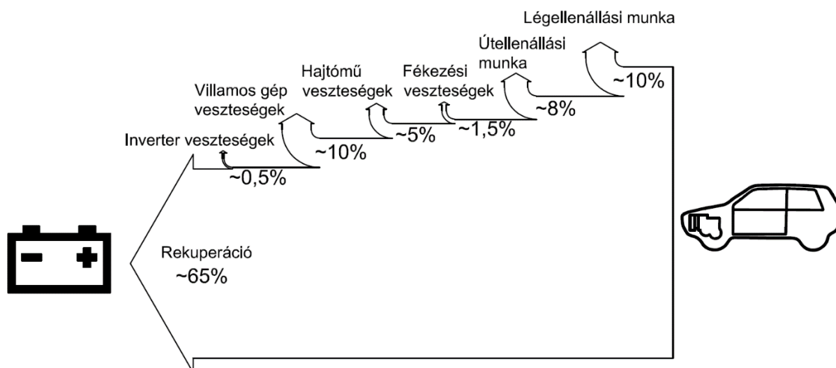
10. ábra A példaként alkalmazott elektromos jármű energiamérlege egyenletes lassítás közben
