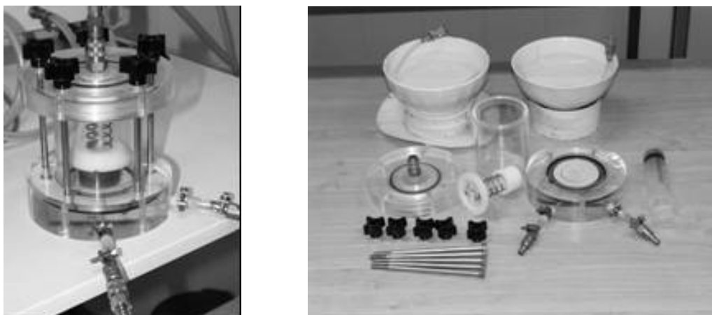
5. ábra A feszültségkamrás készülék
