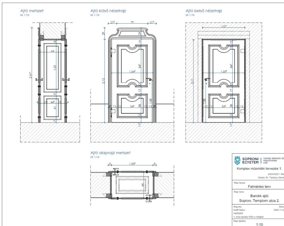
3. ábra. Az emeleti barokk ajtó felmérési rajza (Klaffl Gábor felmérése)
