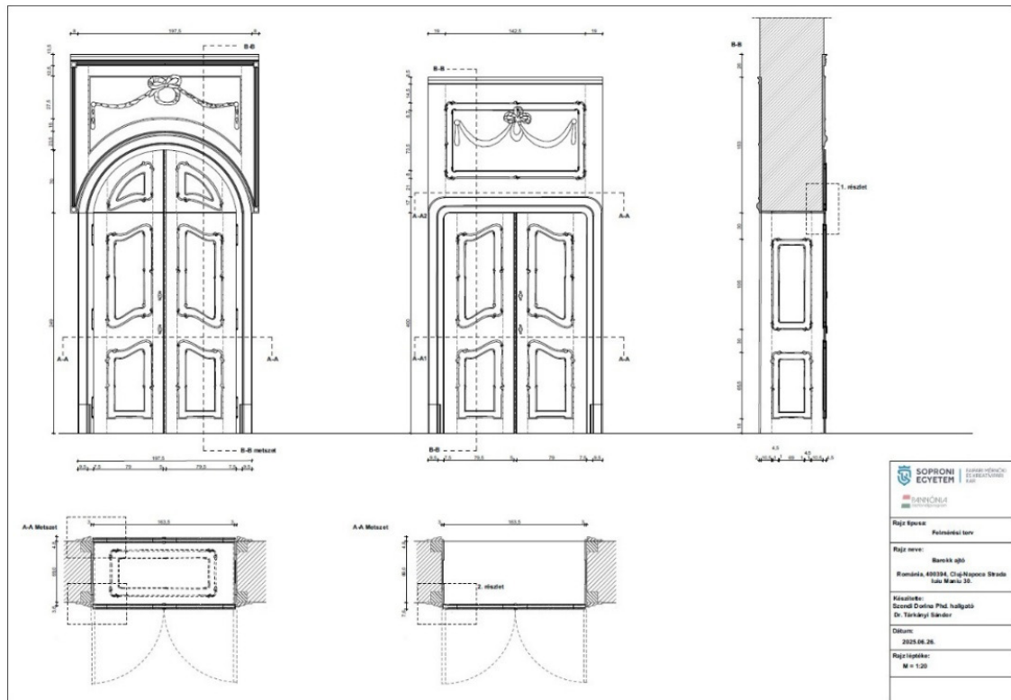
5. ábra. A Bánffy-palota supraportos kétszárnyú ajtajának felmérési rajza (Szendi Dorina felmérése)
