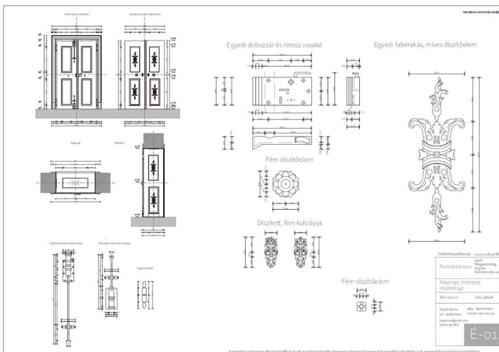
4. ábra. Az emeleti porcelánkabinet kétszárnyú ajtajának felmérési rajza (Bognár Bianka felmérése)
