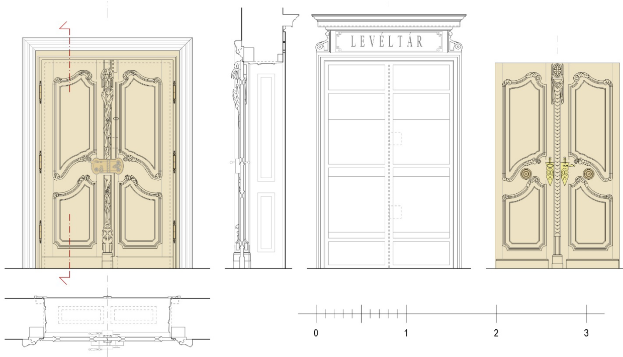
5. ábra. A Levéltár ajtajának felmérési rajza [8]
