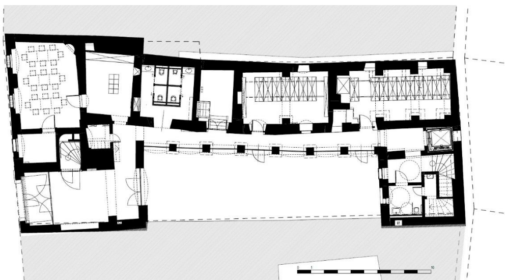
2. ábra. A Sopron, Templom utca 17. számú barokk épületben kialakított könyvtár megvalósult földszinti alaprajza [6]
