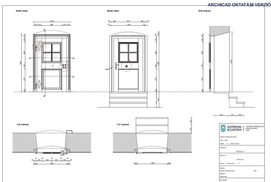
3. ábra. A földszinti, üvegezett barokk ajtó rajza (Németh-Zsuppányi Patrik felmérése)
