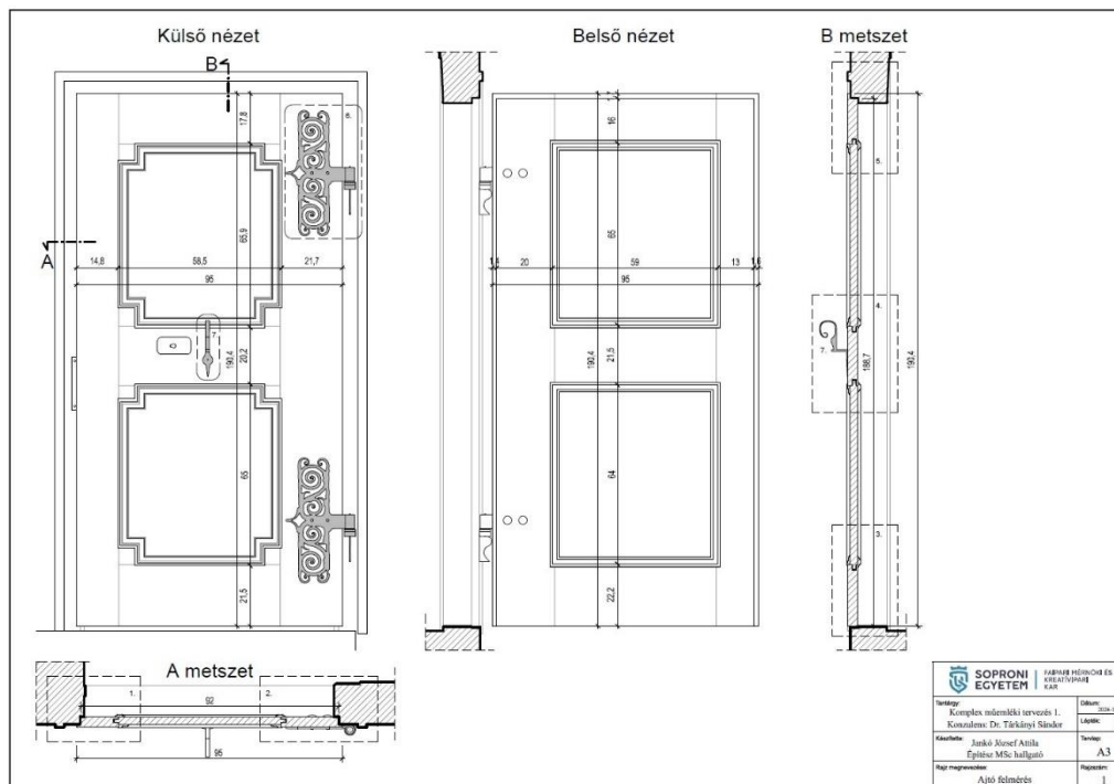
3. ábra. A földszinti barokk ajtó rajza (Jankó József Attila felmérése)
