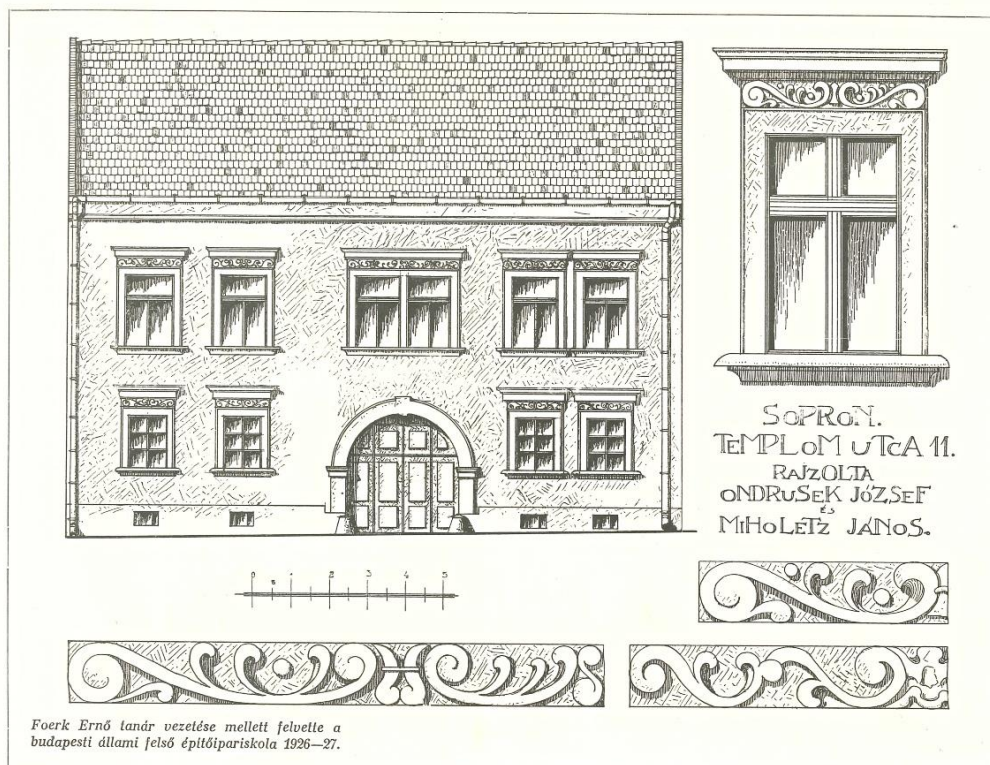
2. ábra. A Sopron, Templom utca 11. számú barokk lakóház homlokzatának és kőfaragványainak 1926-27-es felmérési rajza [4]
